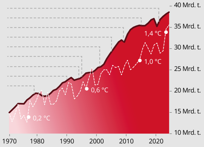
Daten: Met Office Hadley Centre 2026 and Global Carbon Project 2025
